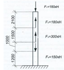
Расчетная схема стойки М 1:100
