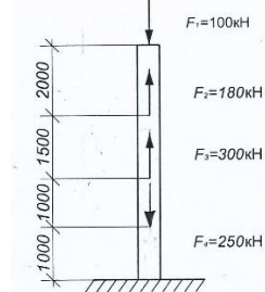
Расчетная схема стойки М 1:100
