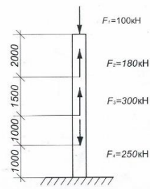
Расчетная схема стойки М 1:100
