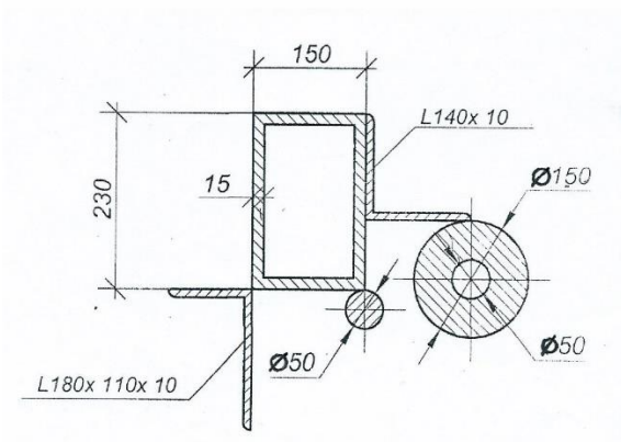
Сложное сечение М 1:100
