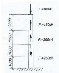
Расчетная схема стойки М 1:100
