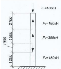
Расчетная схема стойки М 1:100
