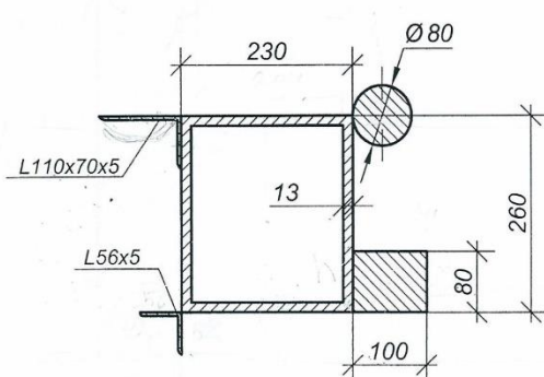
Сложное сечение М 1:100
