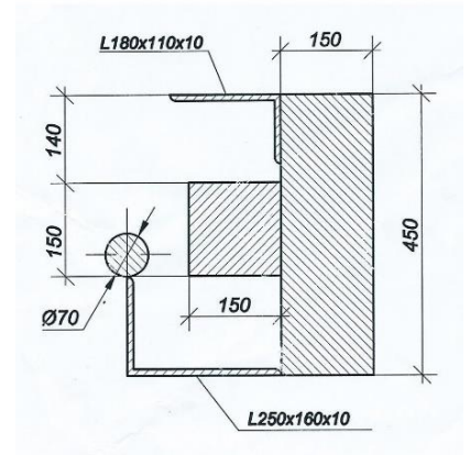
Сложное сечение М 1:100
