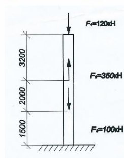
Расчетная схема стойки М 1:100
