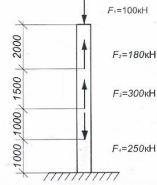
Расчетная схема стойки М 1:100
