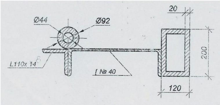
Сложное сечение М 1:100
