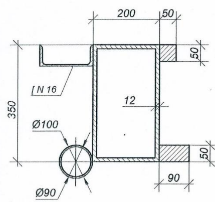
Сложное сечение М 1:100
