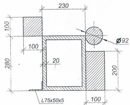
Сложное сечение М 1:100
