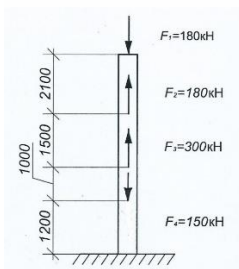
Расчетная схема стойки М 1:100
