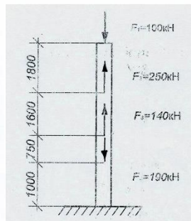
Расчетная схема стойки М 1:100
