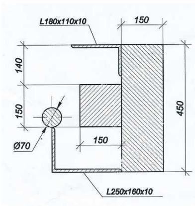
Вариант 10 Сложное сечение М 1:100
