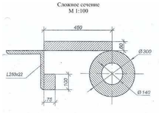
Вариант 9 Сложное сечение М 1:100
