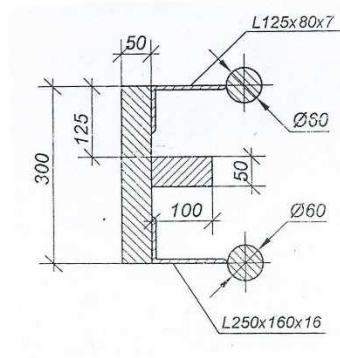
Сложное сечение М 1:100
