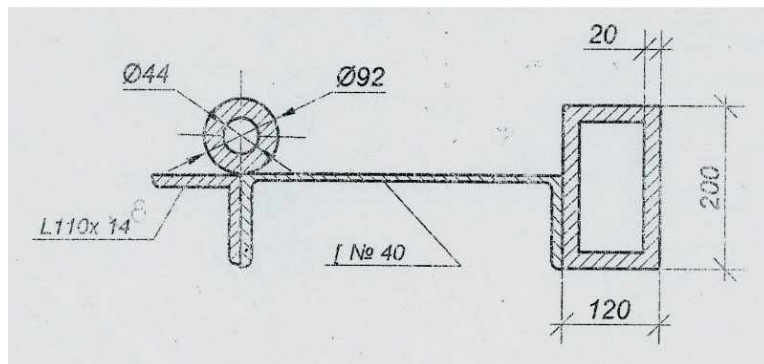
Вариант 9 Сложное сечение М 1:100
